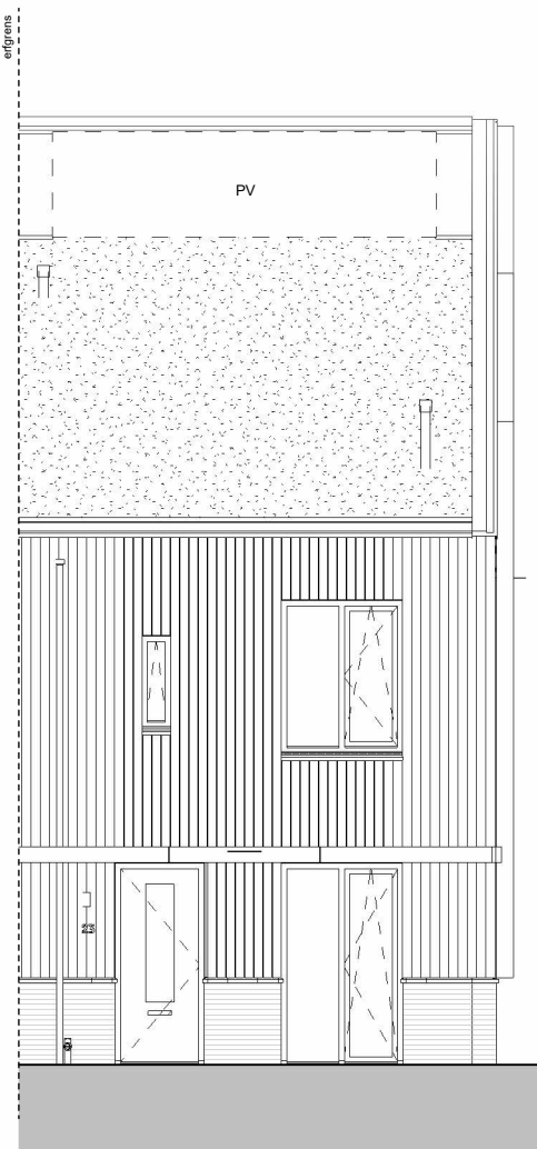
voorgevel
