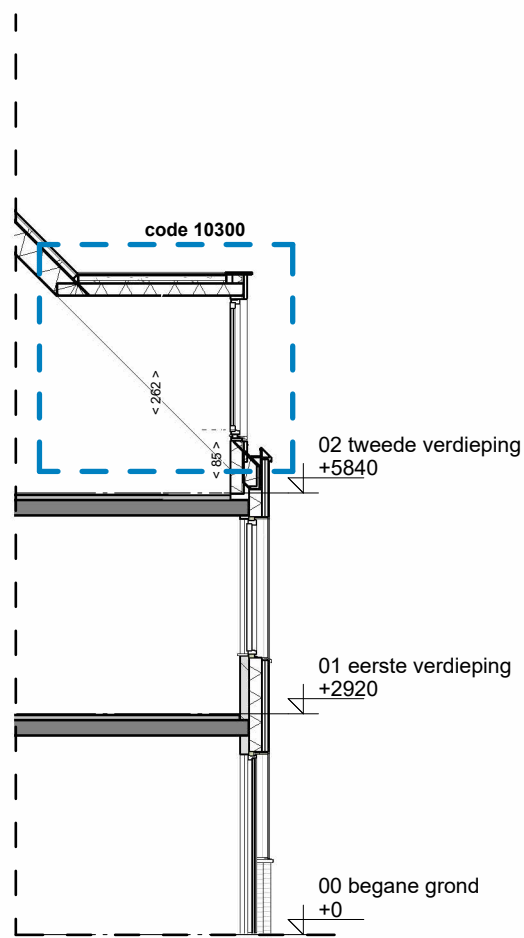
doorsnede
